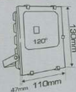
Pha LED 005 10W ●● Kích thước: 110x130xH47 Quang thông: 1020Lm Góc chiếu: 120° 420.000
